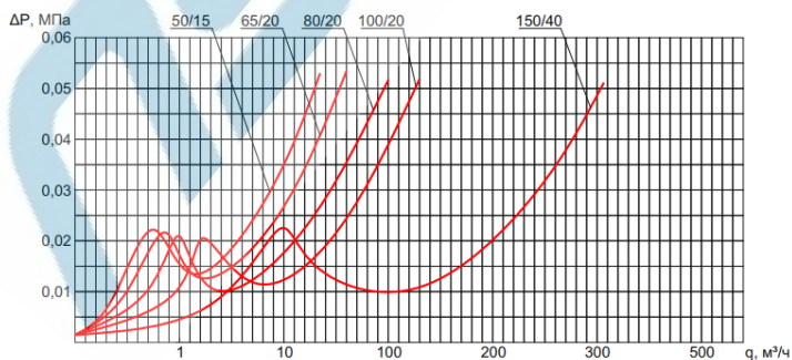
Диаграмма потери давления
