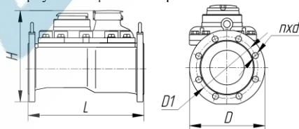
Корпус со встроенным крыльчатим счетчиком
