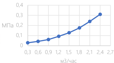
График потери давления
