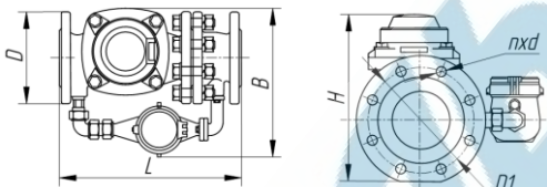
Корпус с выносным крыльчатим счетчиком
