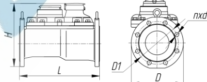
Корпус со встроенным крыльчатим счетчиком
